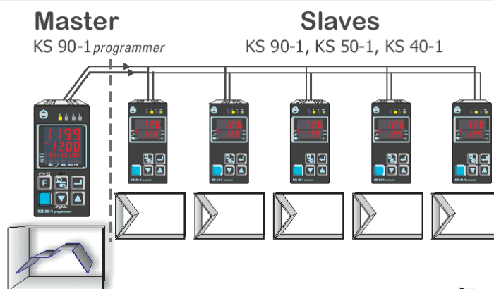
Modbus主控制器发出设定点信号至从控制器
