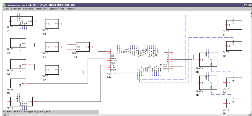
Fig. 2 Operating display for a controller (CONTR, CONTR+)
