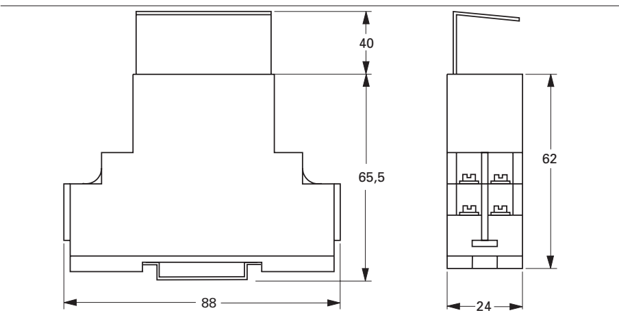
Fig. 1 Dimensions (mm)
